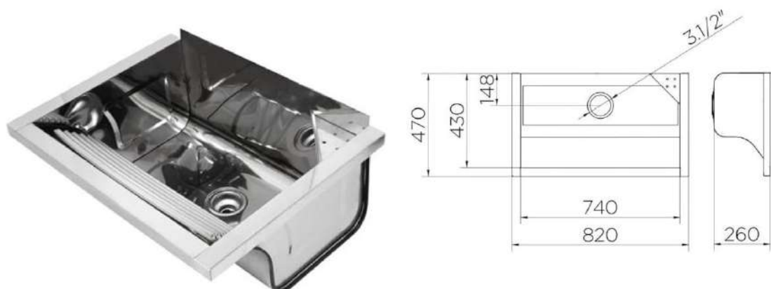
Figura 10 – Tanque reto em aço inox Docol 47 litros.
