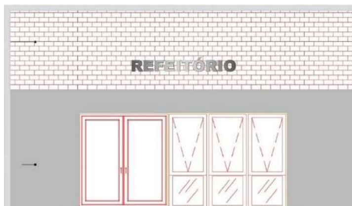
Figura 4 – Vista frontal P04 (porta com painel de vidro adjacente).
