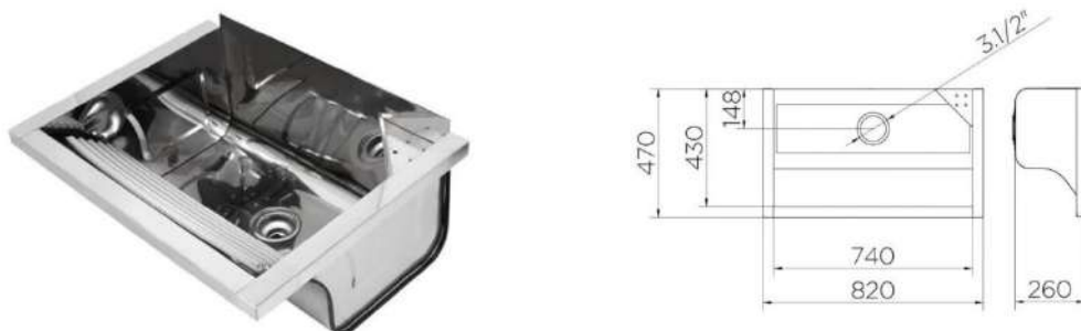
Figura 11 – Tanque reto em aço inox Docol 47 litros.
