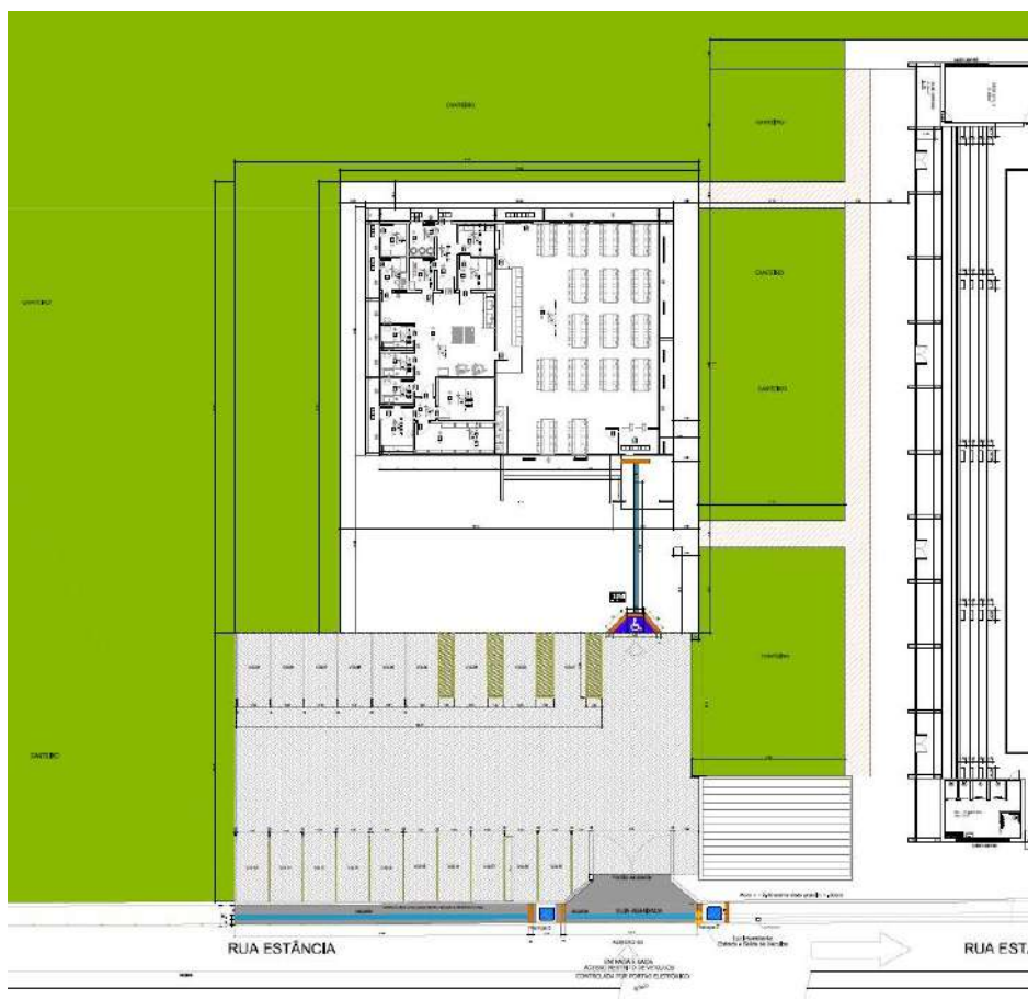
Figura 2 – Locação do Restaurante no campus Aracaju.
