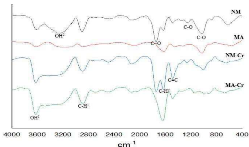
Figura 1 - FTIR das amostras NM e MA sem e com adsorção ao Cr(VI): NM, MA, NM-Cr e MA-Cr. Analisados na região de 400–4000 \text{cm}^{-1} . Nota: \text{OH}^1 – Álcoois e fenóis – livres; \text{OH}^2 – Álcoois e fenóis – ligações de H / Ácidos carboxílicos; \text{C-H}^1 – Alcanos (estiramentos) / Aldeídos; \text{C=O} – Éster / Ácido carboxílico; \text{C=C} – Alceno / Aromático; \text{C-H}^2 – Desdobramento \text{CH}_3 e \text{CH}_2 de alcanos; \text{C-O} – Álcoois, éteres, ésteres, ácidos carboxílicos e anidridos.
