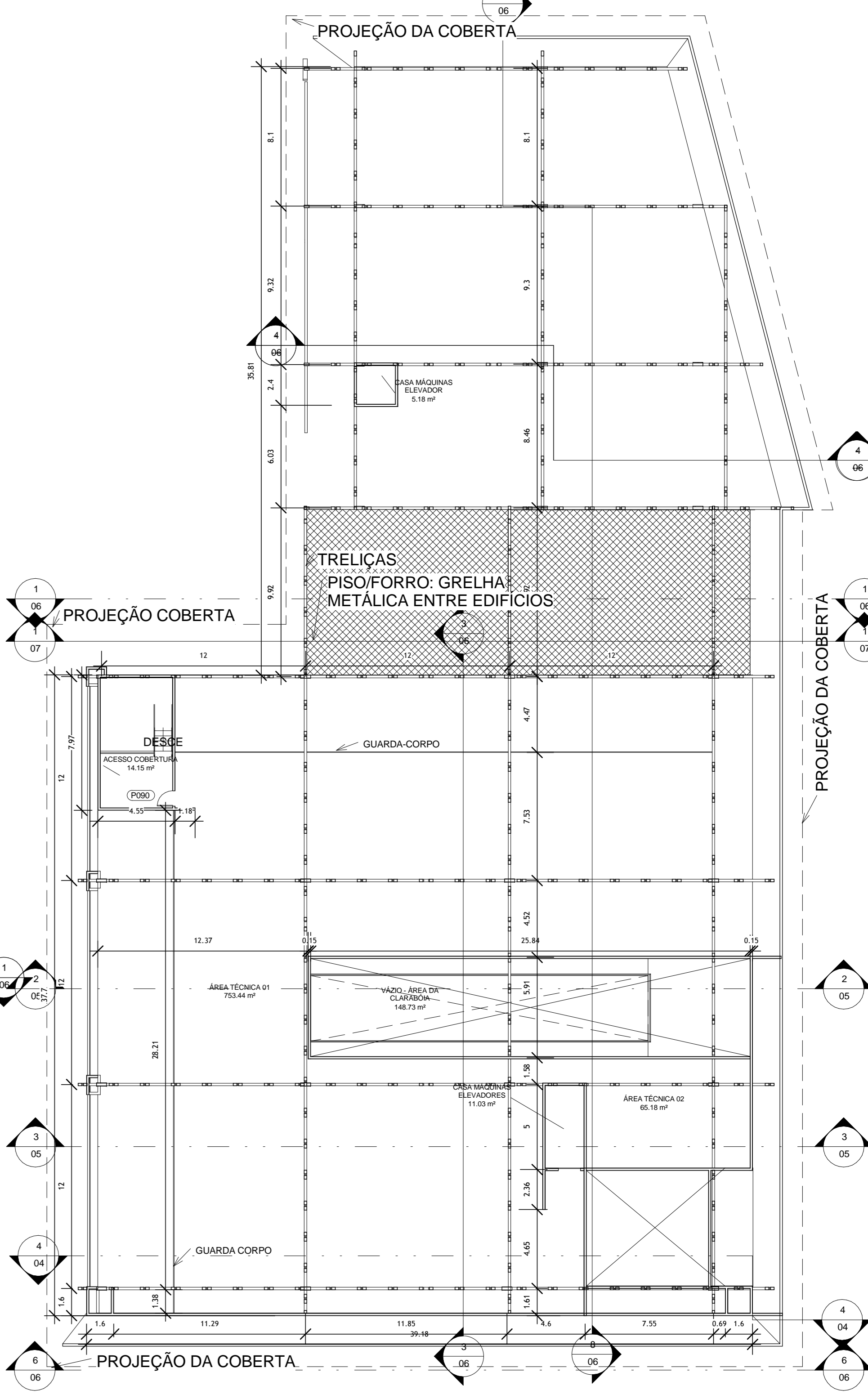
NV.16,00 - 5º PVTO - ESTRUTURA DA COBERTA
